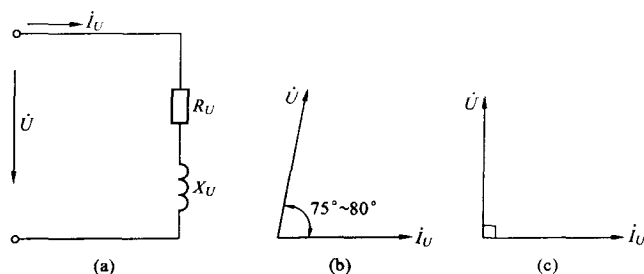
图 2-2 电压电磁铁的等值电路图和相量图
