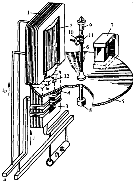
图 2-1 单相电能表的测量机构简图
