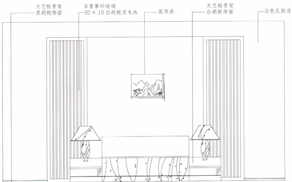
▲ 主卧 B 立面图
