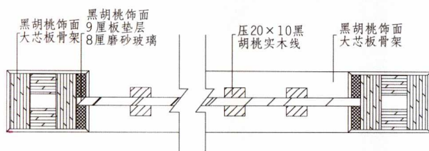
▲ B-B 剖立面图
