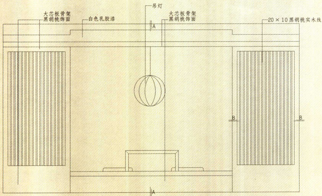
▲ 客厅 D 立面图
