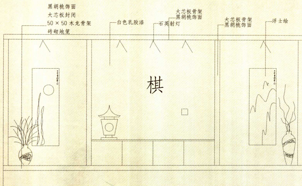
▲ 和室 D 立面图
