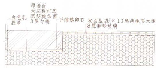
▲ B-B 剖立面图
