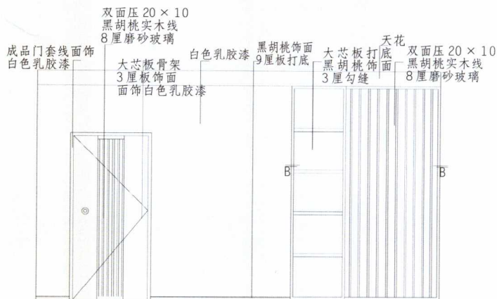
▲ 玄关及门立面图
