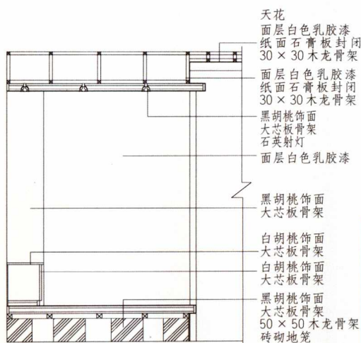
▲ A-A 剖立面图
