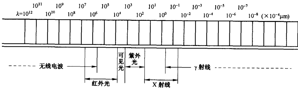
图 1-2 电磁波谱
