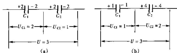
图 1-1-4 双层介质中电荷和电位分布
