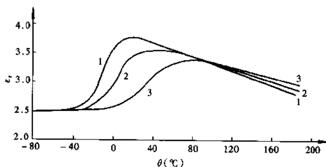
图 1-2-3 硫化天然橡胶的相对介电常数与温度、电场频率的关系
