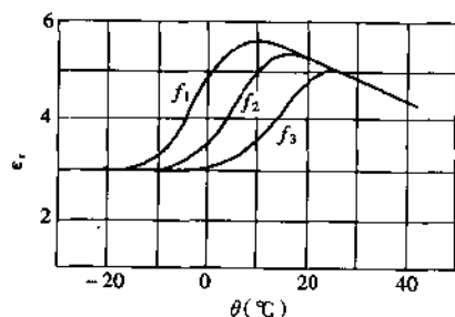
图 1-2-1 氯化联苯的相对介电常数与温度的关系 (频率 f_3 > f_2 > f_1 )
