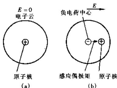
图 1-1-1 电子位移极化
