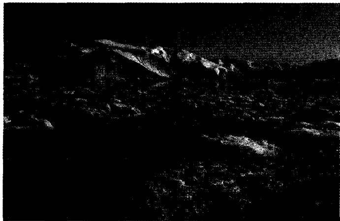
正在融化的 南极冰川
