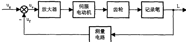
图1.3 例1.1自动记录仪方框图
