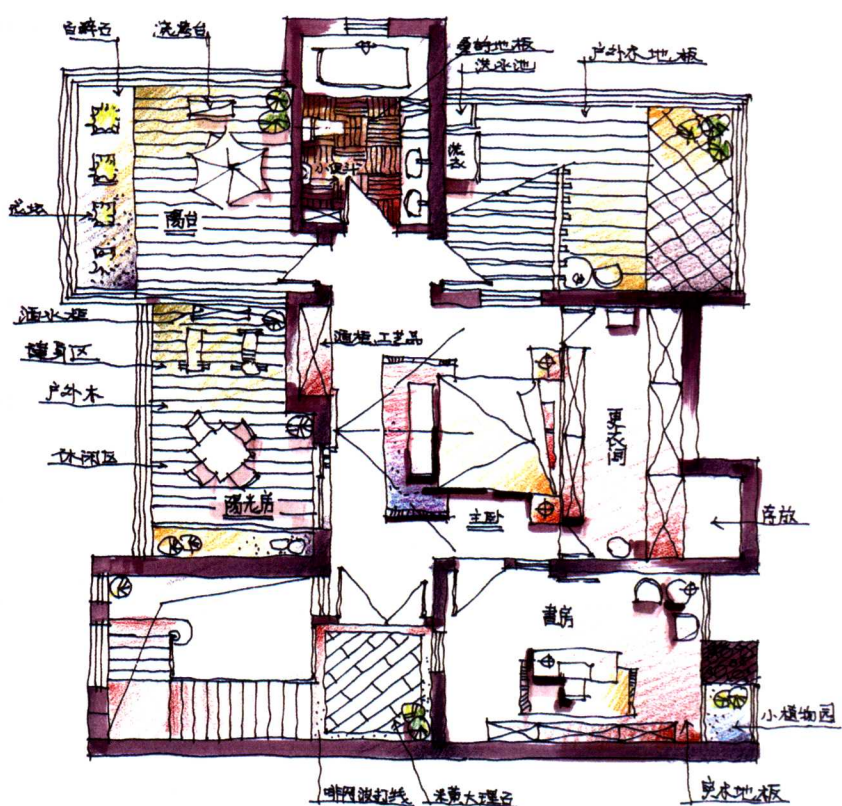
水岸星城雅舍一樓平面布置图 1:75
