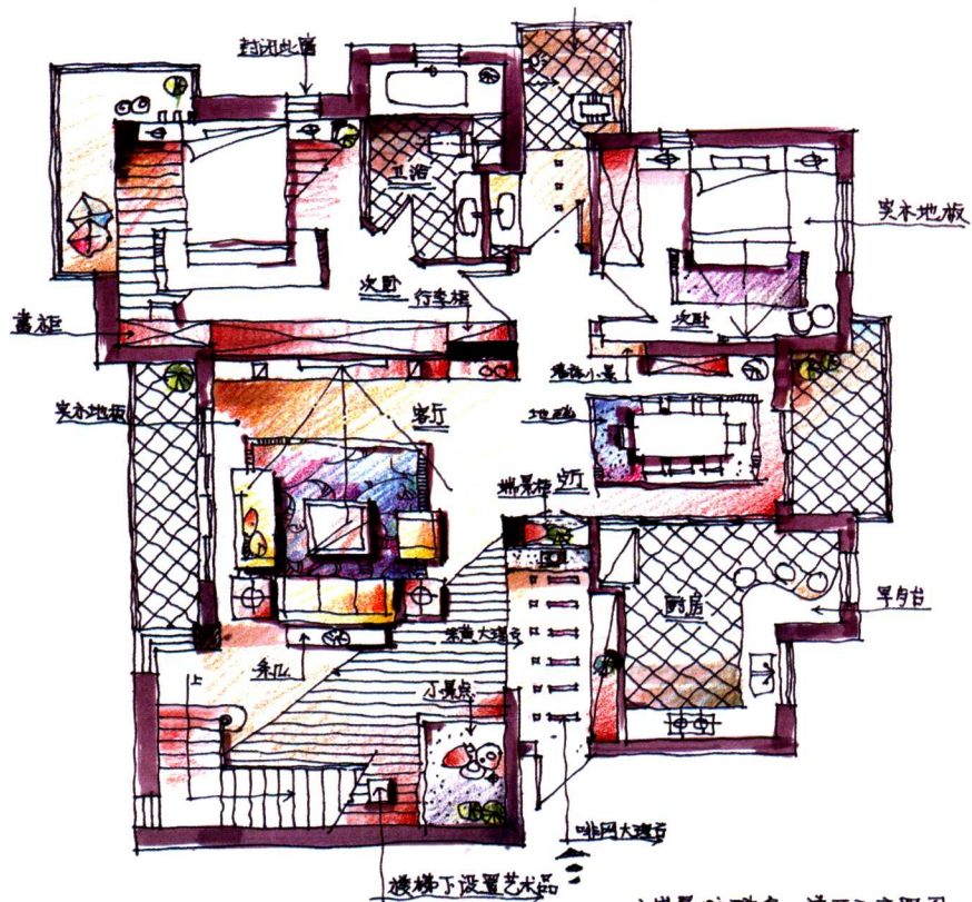
水岸星城雅舍一樓平面布置图 1:75
