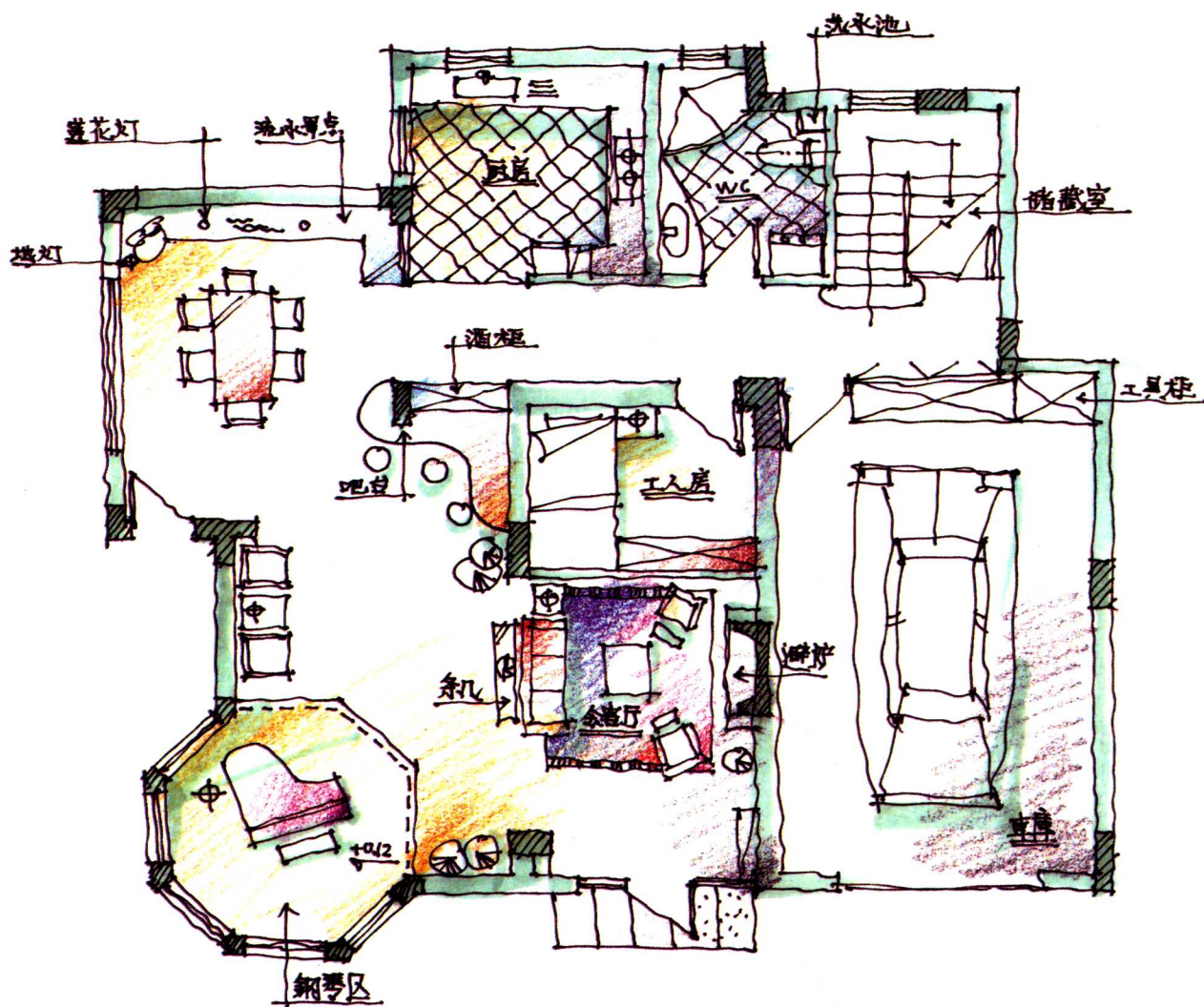
东湖林语别墅一层平面
