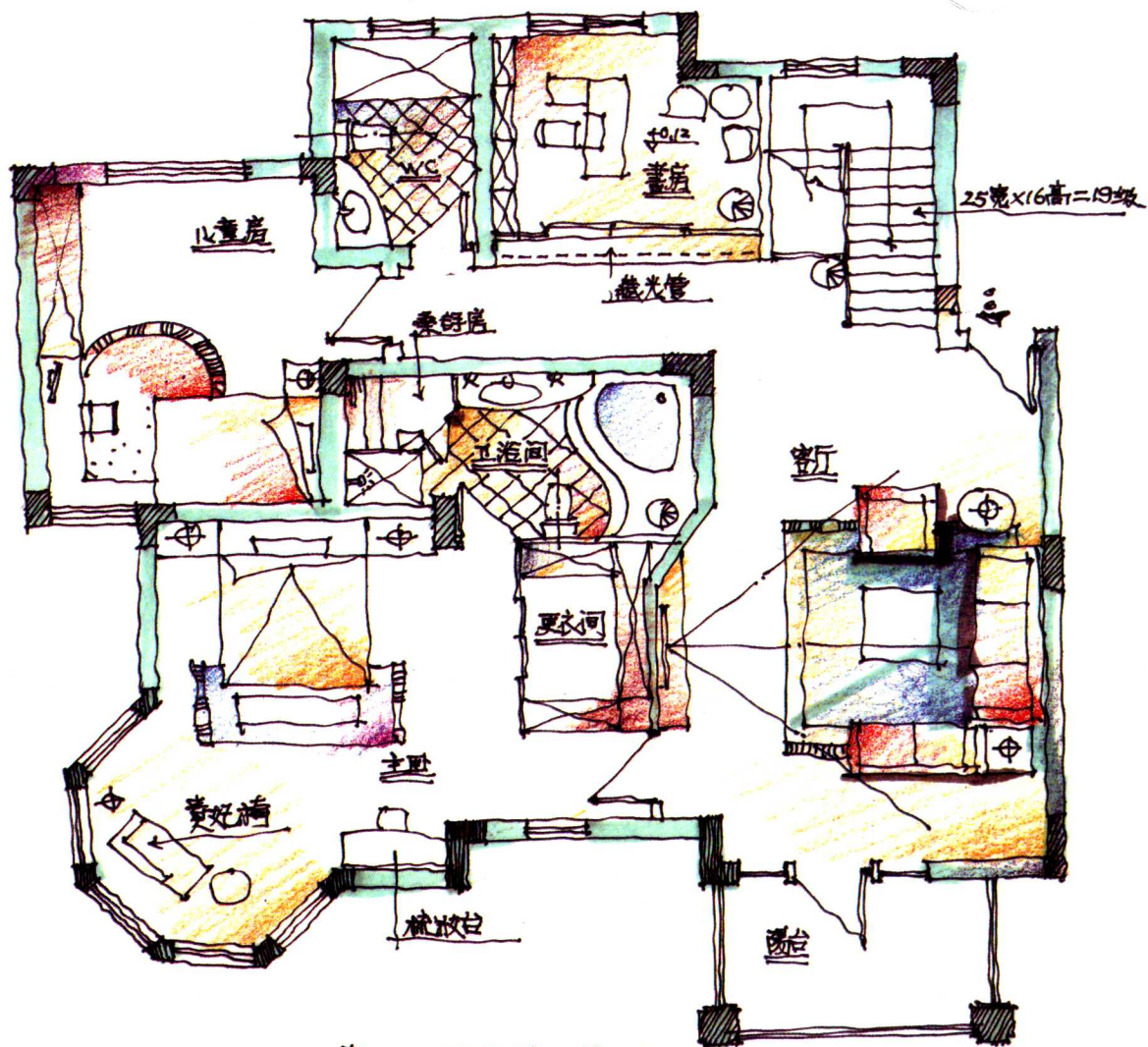
东湖林语别墅二层平面
