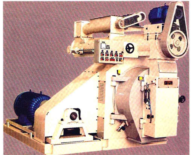
6. 制粒机(型号 PCM)
