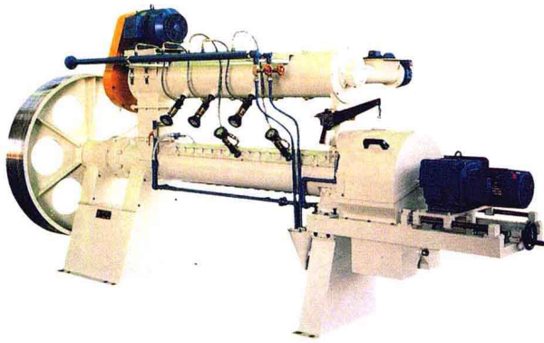
4. 挤压膨化机(型号 ES)
