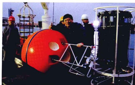
12月1日，南风科创公司参与开发研制的6000米潜标系统成功布放
