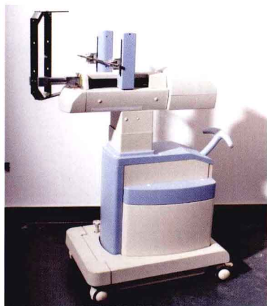
天智航公司研制的骨科导航机器人
