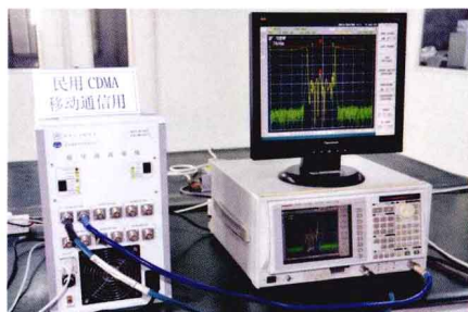
综艺超导科技有限公司研发的 超导滤波系统
