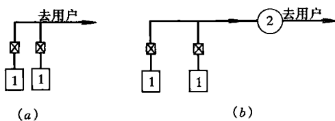
图 1-1-10 低压氧气管道系统 1—分馏塔；2—低压储气器
