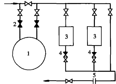
图 1-1-9 低压储存、中压输送储配站工艺流程 1—低压湿式储气罐；2—水封阀门； 3—压缩机；4—止回阀； 5—流量计
