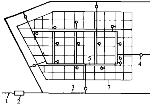
图 1-1-8 高、中、低压三级管网系统 1—长输管线支线；2—门站或配气站；3—高压管网； 4—高、中压调压站；5—中压管网；6—中、低压调压站；7—低压管网
