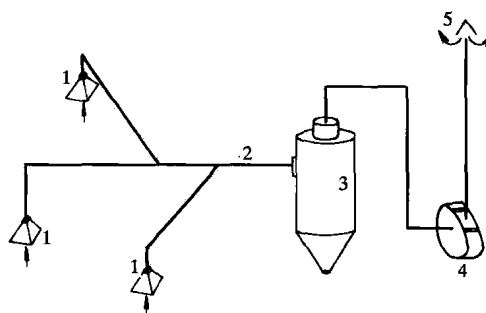
图 1-1-1 排风系统
