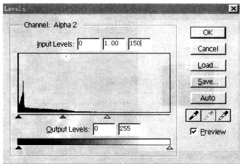
图 1-1-5 Levels 对话框
