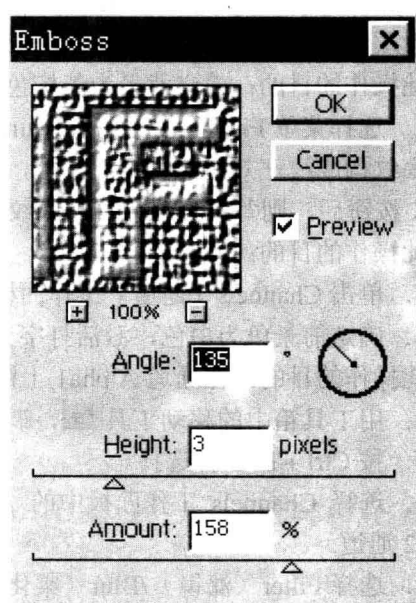
图 1-2-4 浮雕对话框
