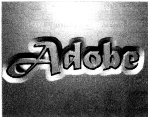
图 1-1-1 制作效果
