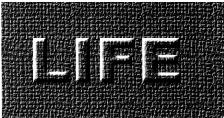
图 1-2-1 图像效果
