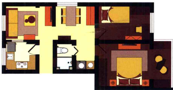
改造后的户型平面图
