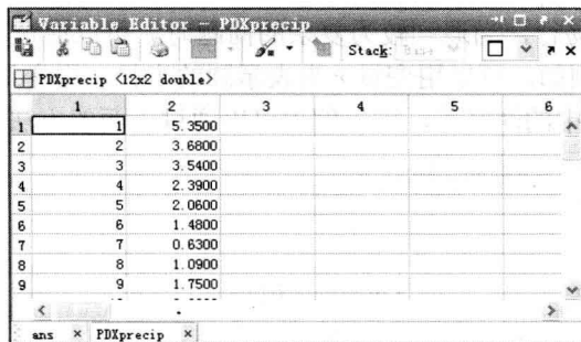
图 1-2 变量编辑器
