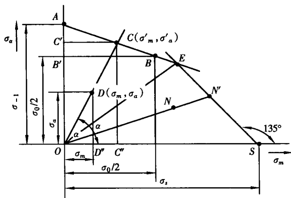
图 1-6 简化的极限应力图
