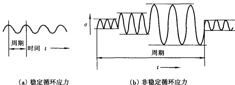
图 1-2 变应力
