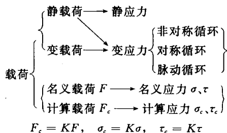
图 1-1 载荷和应力
