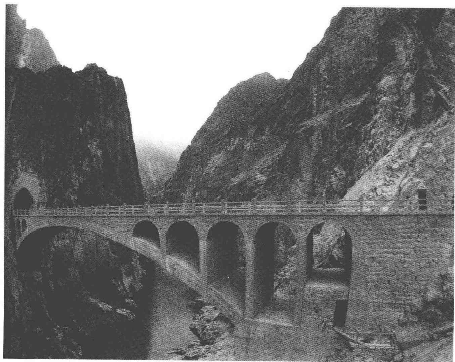
1972年12月29日，怒江大桥改建成钢筋混凝土大桥。
