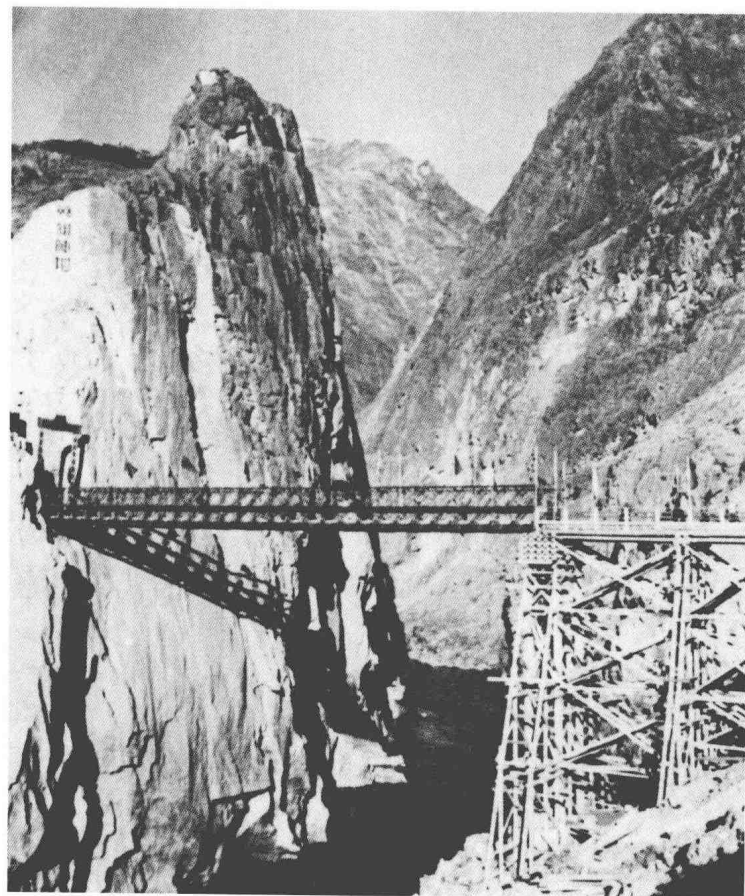
1953年11月1日，在怒江绝壁上建成的贝雷式钢架桥。
