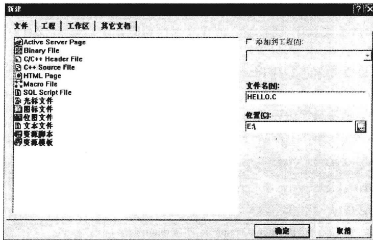
图 1-2 输入文件名
