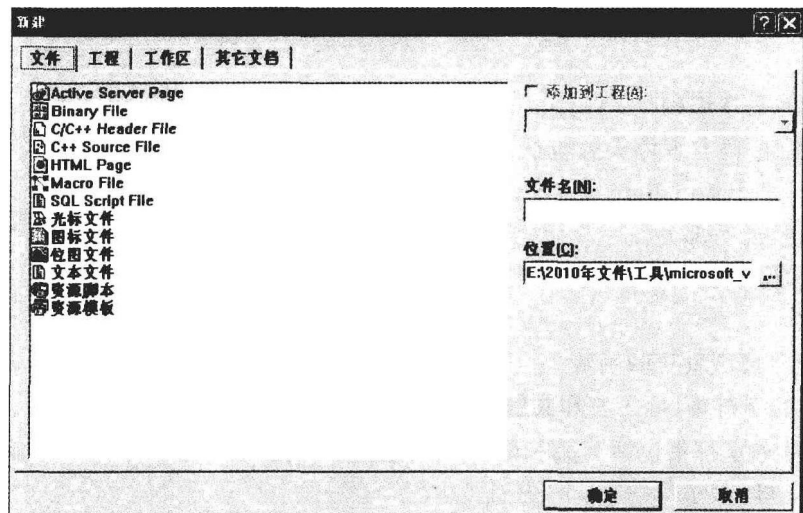
图 1-1 新建窗口
