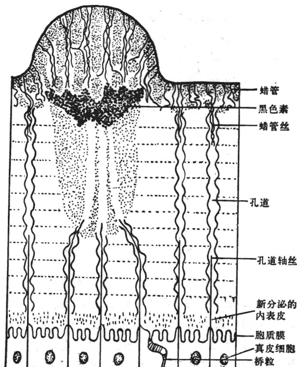
图 11-4 蜡螟幼虫表皮构造(仿 Locke, 1961)
