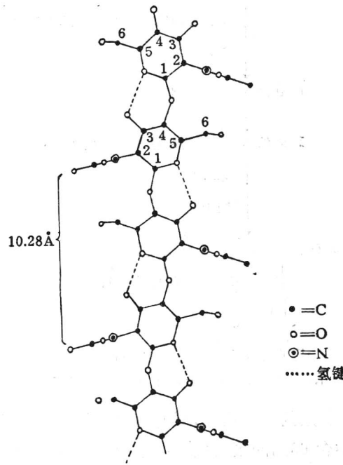
图 11-7 \alpha -几丁质分子结构(仿 Neville, 1967)
