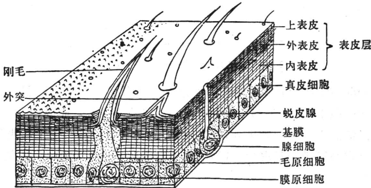
图 11-1 昆虫体壁构造模式图(仿 Richards, 1951)
