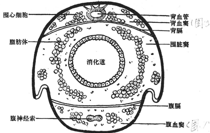
图 §-1 昆虫腹部的横切面(仿 Snodgrass, 1935)
