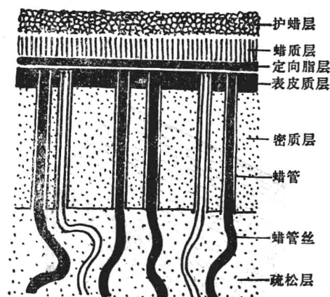
图 11-6 蜡螟幼虫上表皮构造(仿 Locke,1961)
