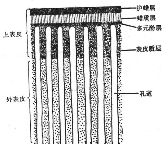
图 11-5 吸血蜡的上表皮构造(依Wigglesworth,1948)
