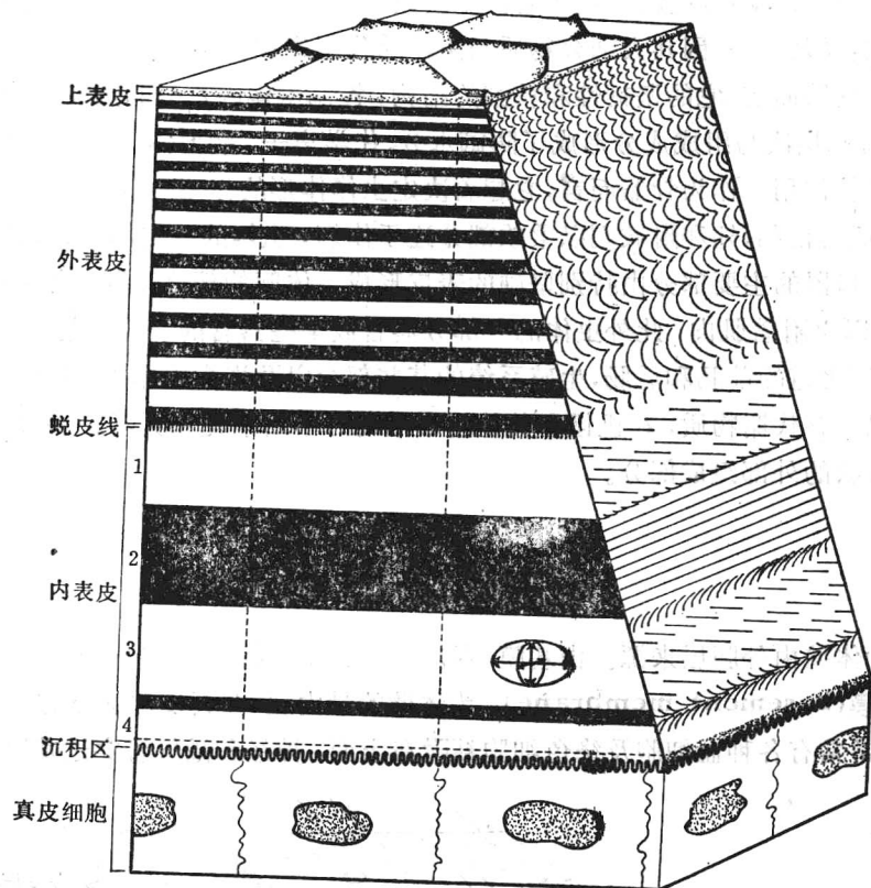
图 11-2 昆虫体壁表皮分层示意图(仿 Caveney,1971)
