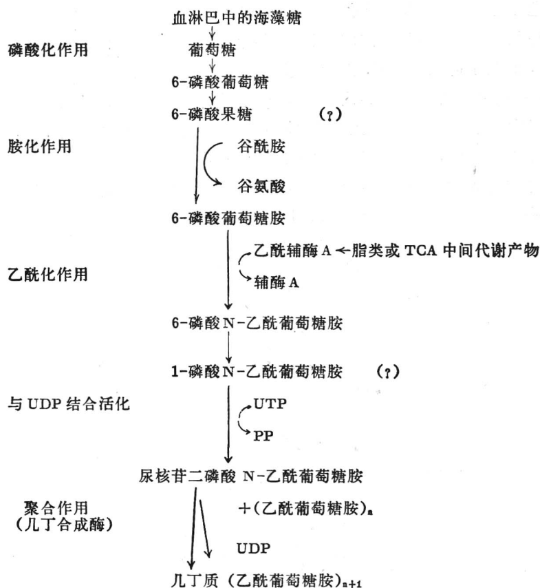
图 11-8 几丁质合成途径(Neville, 1975)
