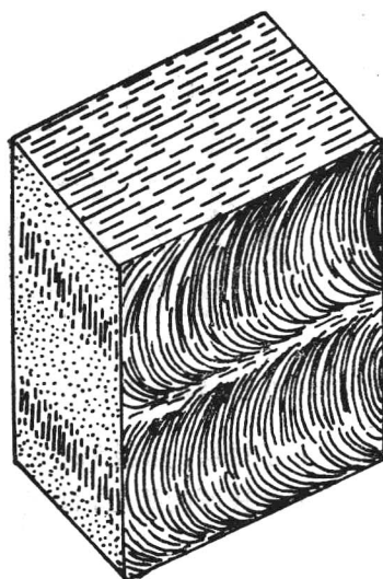
图 11-3 内表皮两个片层的模式图(仿 Bouligand, 1965)
