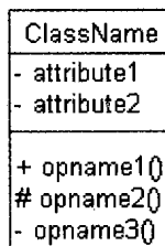
图 1-1 类在 UML 中的表示示例
