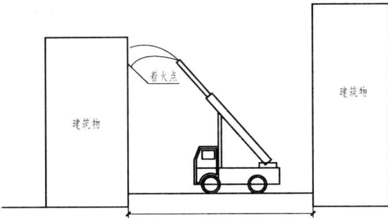
图 1-1-6 防火间距=使云梯展开的宽度+喷水宽度
