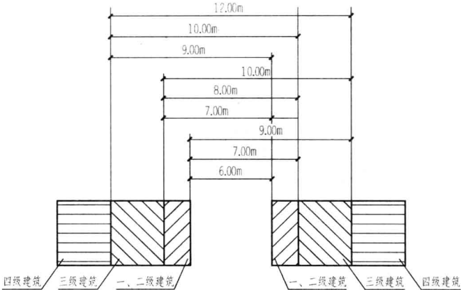
图 1-1-4 民用建筑之间的防火间距
