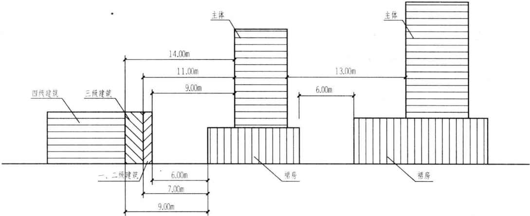
图 1-1-5 高层建筑之间及高层建筑与其他民用建筑之间的防火间距
