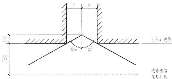
图 1-2-1 汽车库库址车辆出入口通视要求
