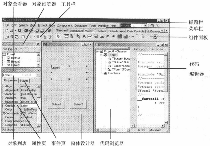
图 1-1 C++ Builder 6 的 IDE 主界面
