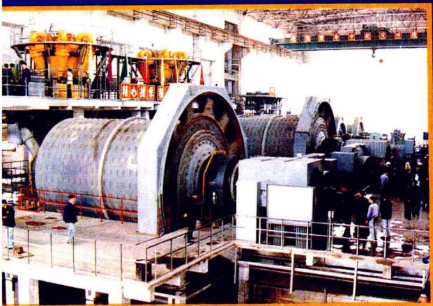
江西永平铜矿选矿厂 5×6.4 米加拿大进口球磨机（两台）
