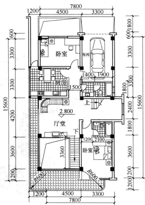
A型二层平面图
