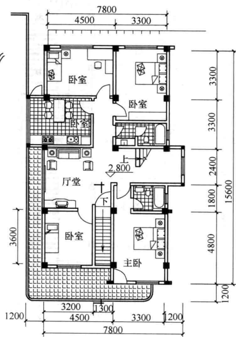
B型二层平面图
