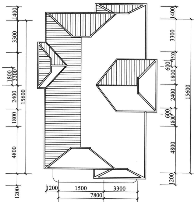
A型屋顶平面图
