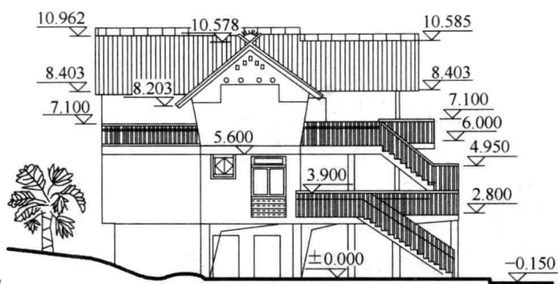
C 型东立面图
