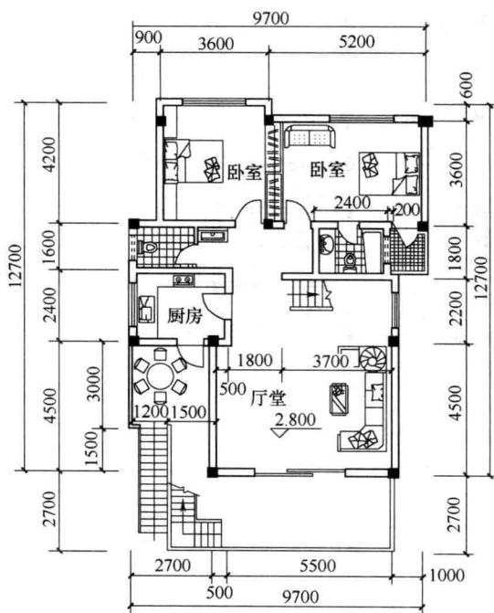
C 型二层平面图
