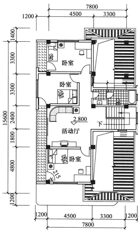
A型三层平面图
