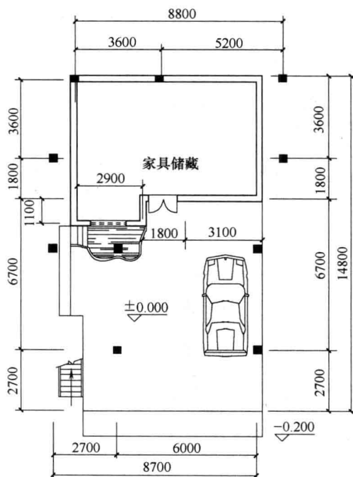
C 型一层平面图
