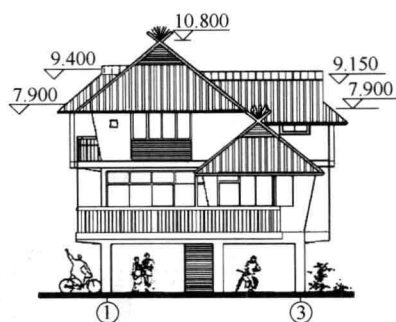
A型南立面图
