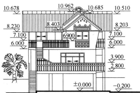
C 型南立面图
