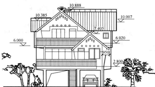
B型南立面图
