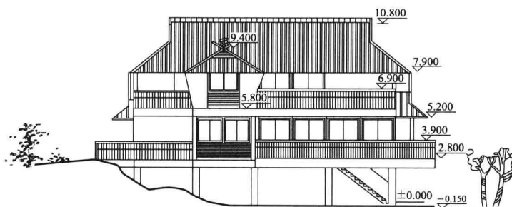
A型东立面图
