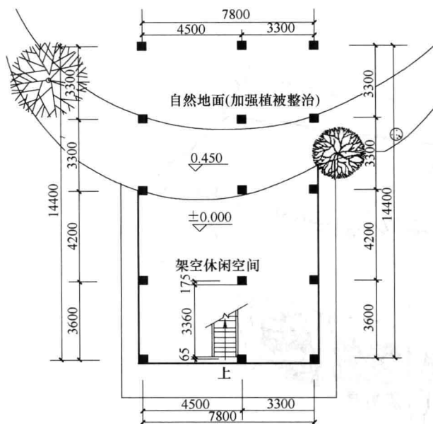
A型一层平面图
