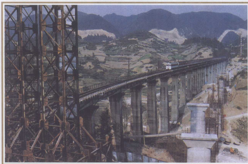
·建设中的株六(株州——六盘水)复线工程的重中之重——新马拉特铁路桥(赵帆 摄)
