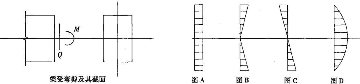
截面剪应力分布图
