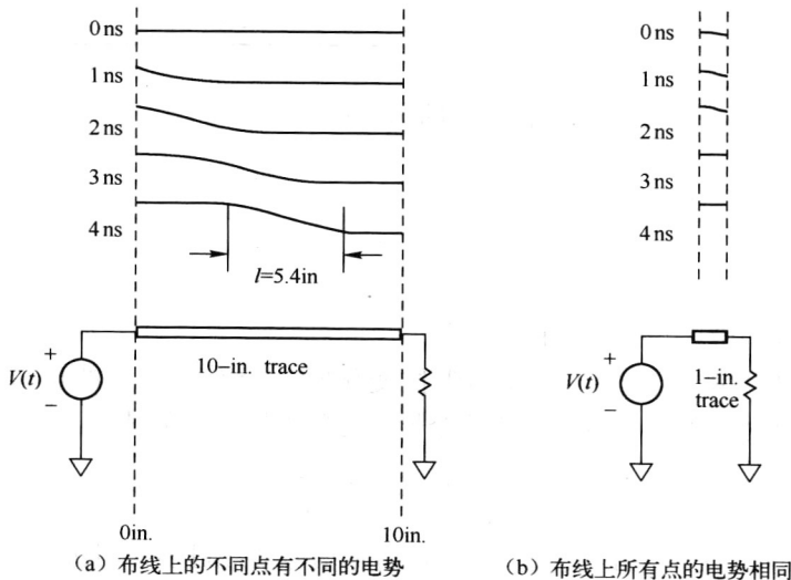
图 1-3-2 两种信号布线
