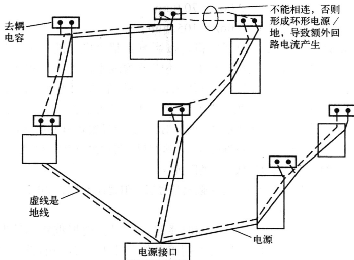
图 1-3-8 较好的单面板设计
