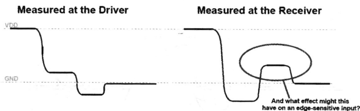
图 1-3-5 示波器观察结果
