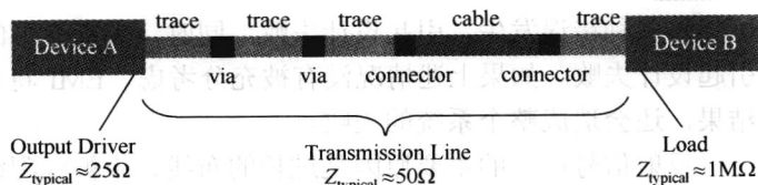
图 1-3-4 信号传输路径
