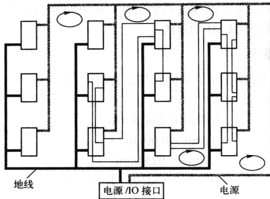
图 1-3-7 较差的单面板设计
