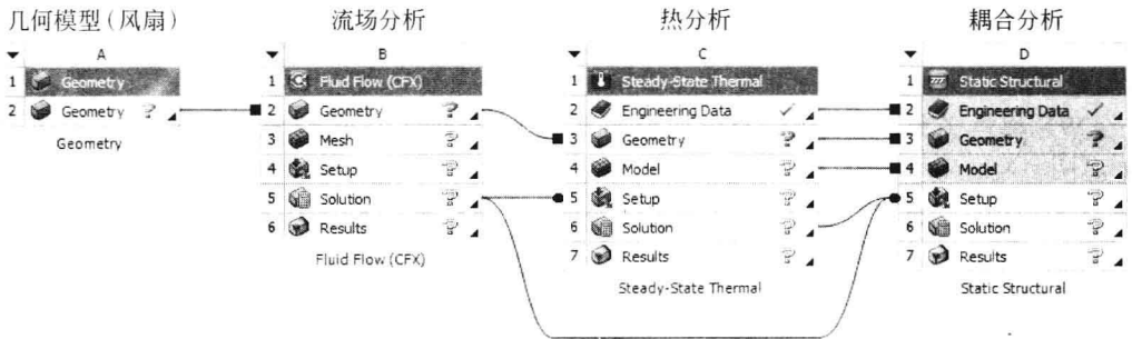
图 1.2 典型叶片流固热耦合分析流程图
