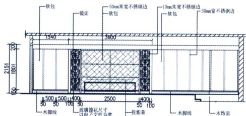
④三层影视室D立面图
