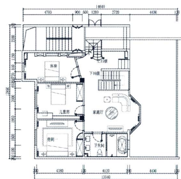
二层平面布置图
