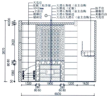
C 客厅电视背景造型立面图
