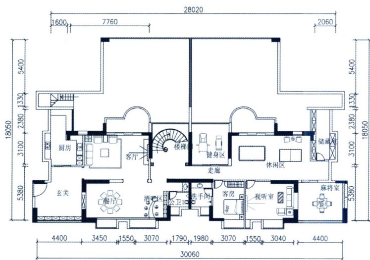
一层平面布置图
