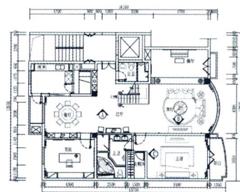
首层平面布置图
