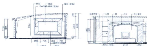
⑤三层影视室E立面图
