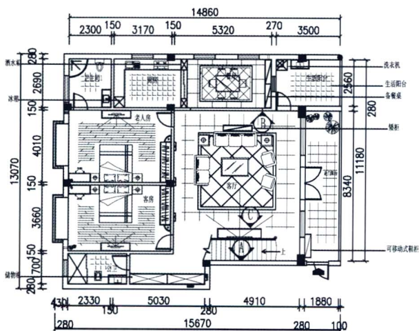
一层平面布置图
