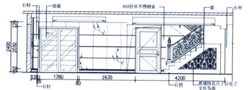
⑦餐厅A立面图
