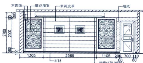
③主卧C立面图
