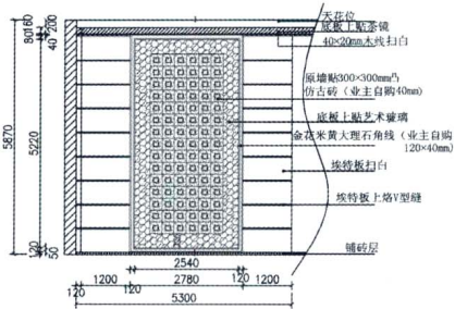
A 客厅楼梯墙面背景造型立面图
