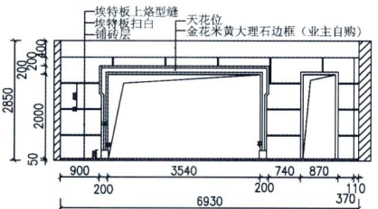
B 墙面及厨房门廊造型立面图
