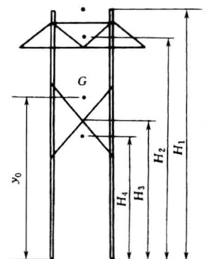
图 1-7 \Pi 型混凝土杆架重心的高度
