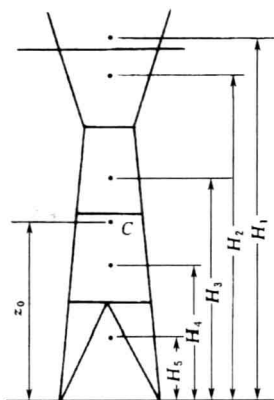
图 1-8 酒杯型塔风荷中心的高度
