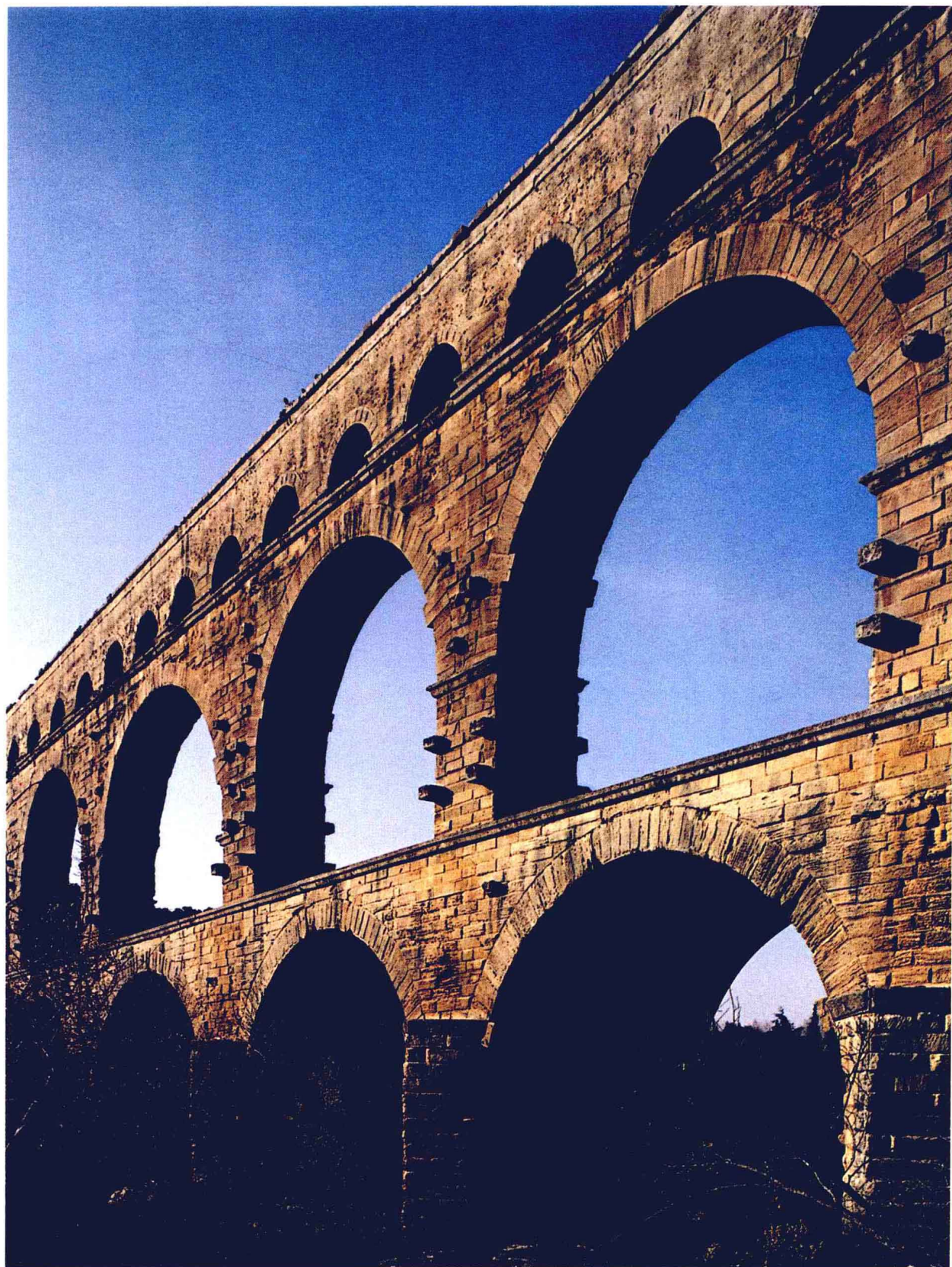
彩图13 引水渠，加尔桥，尼姆，法国（公元1世纪早期）
