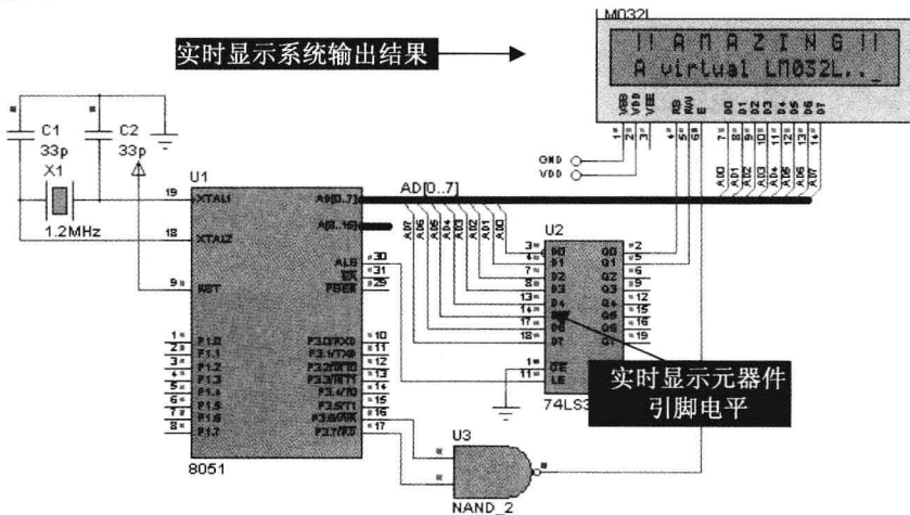
图 1-8 微处理器交互仿真实例
