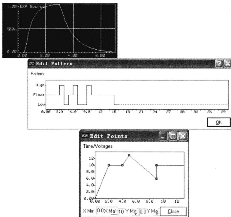
图 1-3 Proteus 激励源的可编辑格式示例
