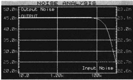
图 1-6 741 放大电路的噪声分析
