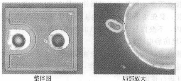
图 1-4 被静电击伤的芯片
