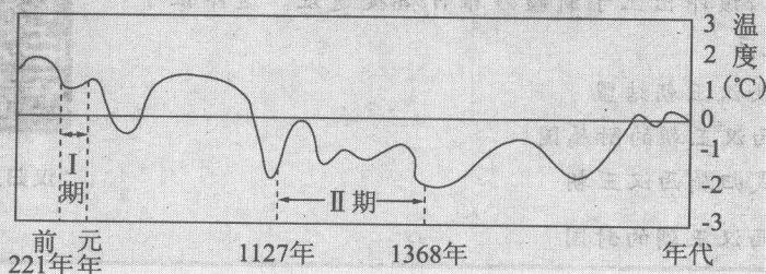
图5 中国2000多年来的气温变化曲线示意图
