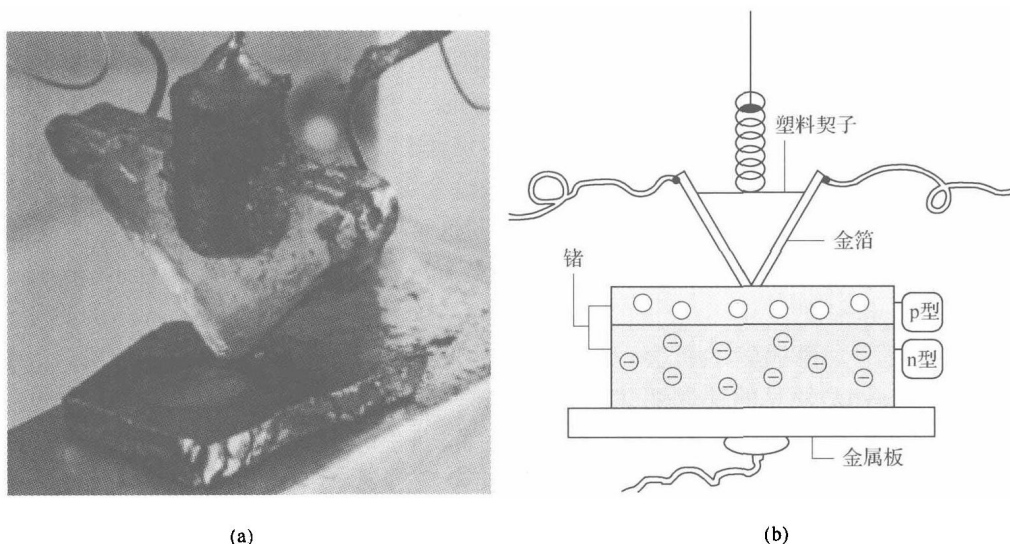
图 1.3 肖克利、巴丁及布拉顿发明的第一个晶体管(a)及其示意图(b)
