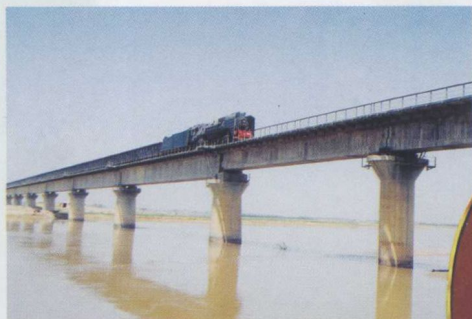
▲ 灵武铁路黄河特大桥，全长1576米，获中国建筑工程鲁班奖
