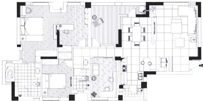
平面布置图
