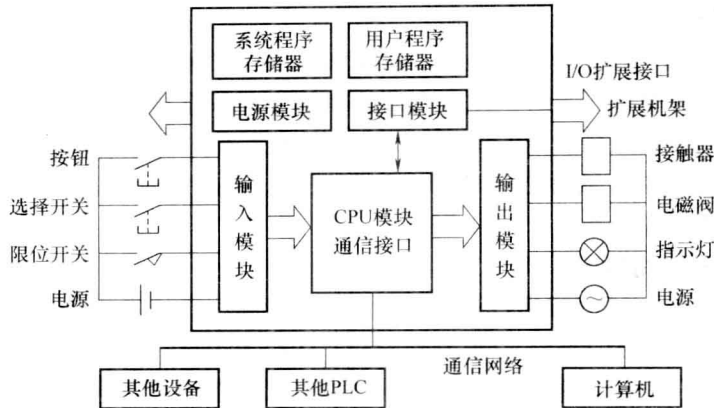
图 1-1 PLC 的组成
