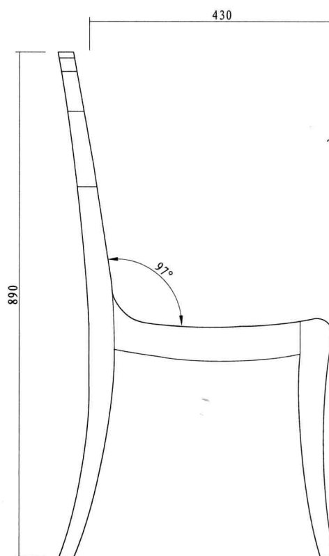
左视图 left view
