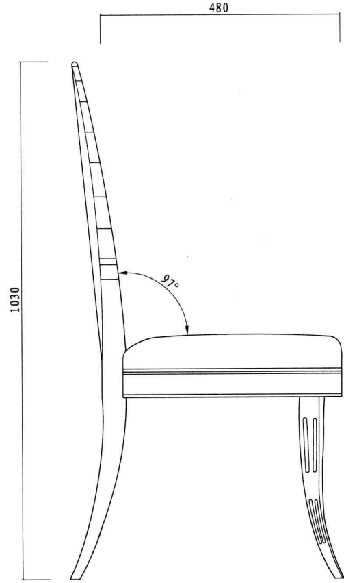
左视图 left view
