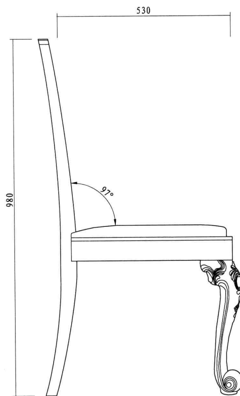
左视图 left view
