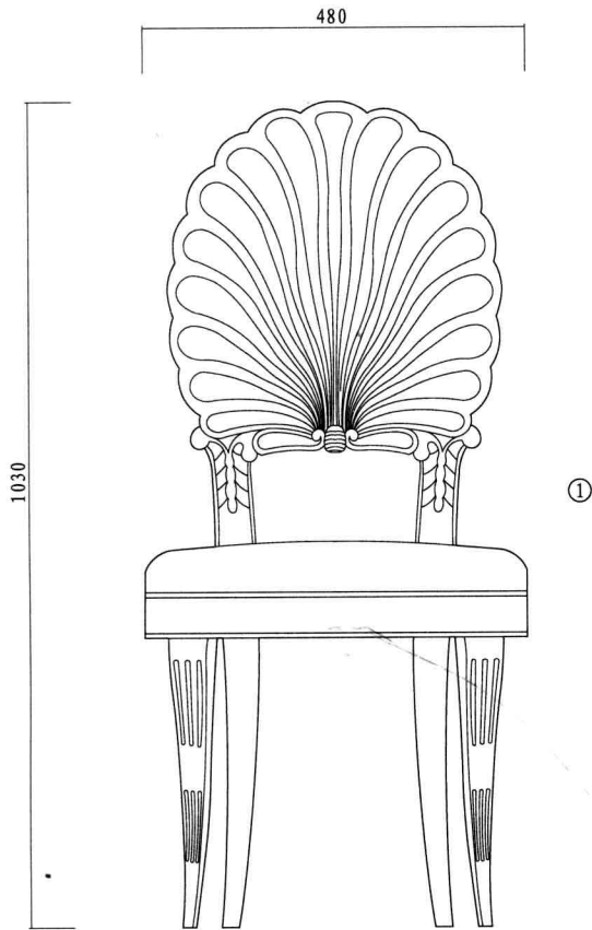
主视图 front view
