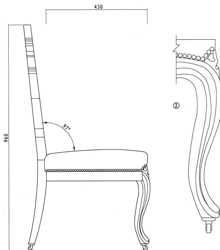
左视图 left view
