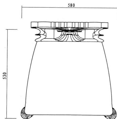
俯视图 top view
