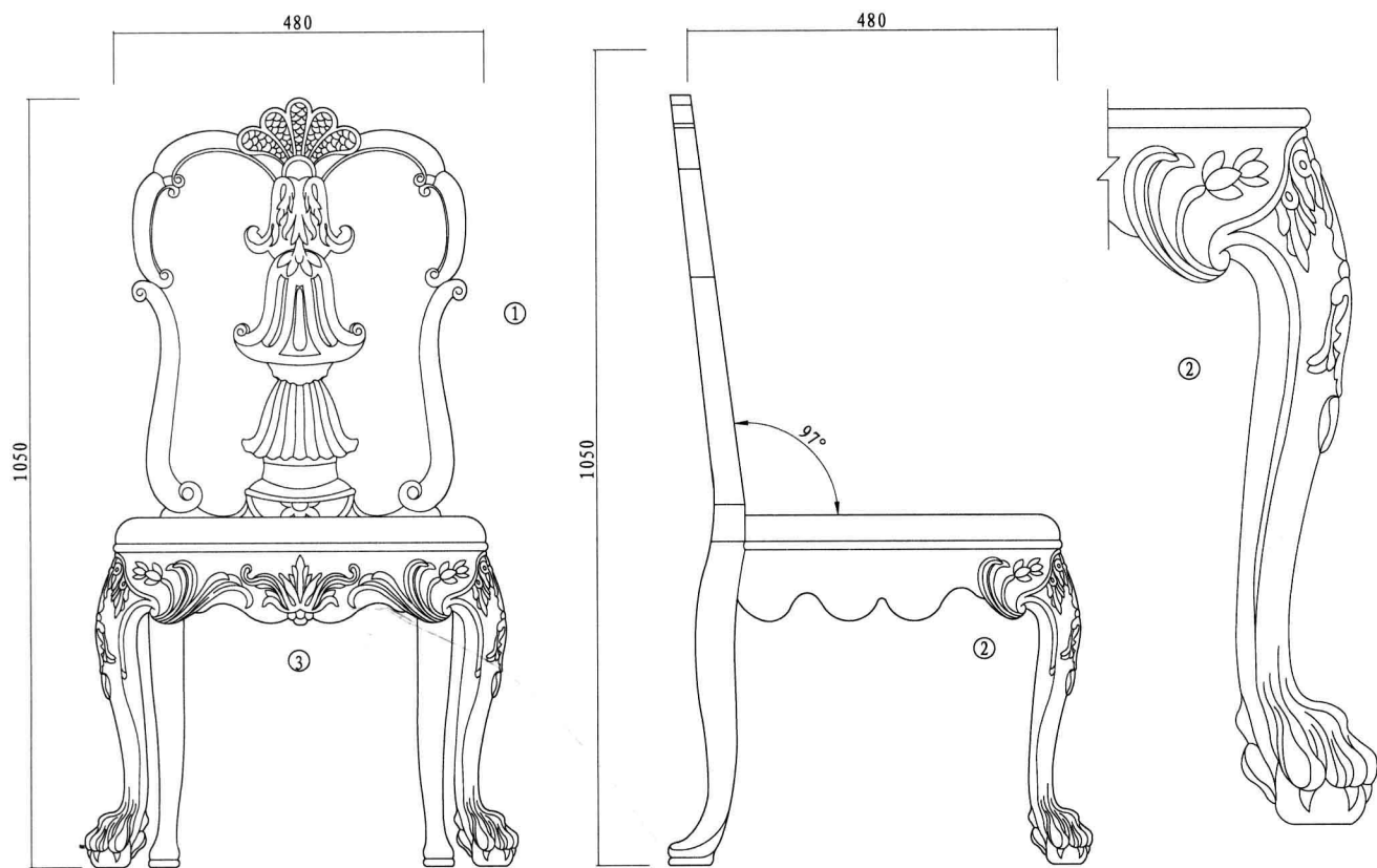
主视图 front view
