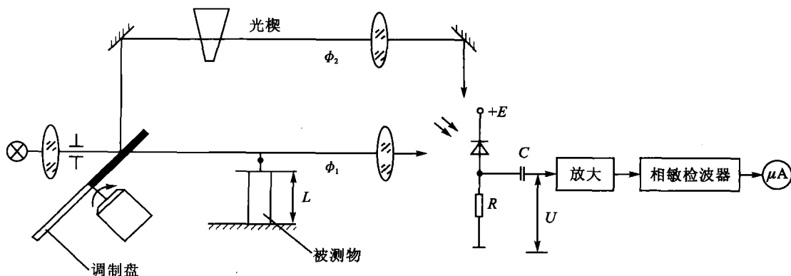
图 1-6 双光路差动测量法测量物体长度
