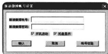
登录界面
