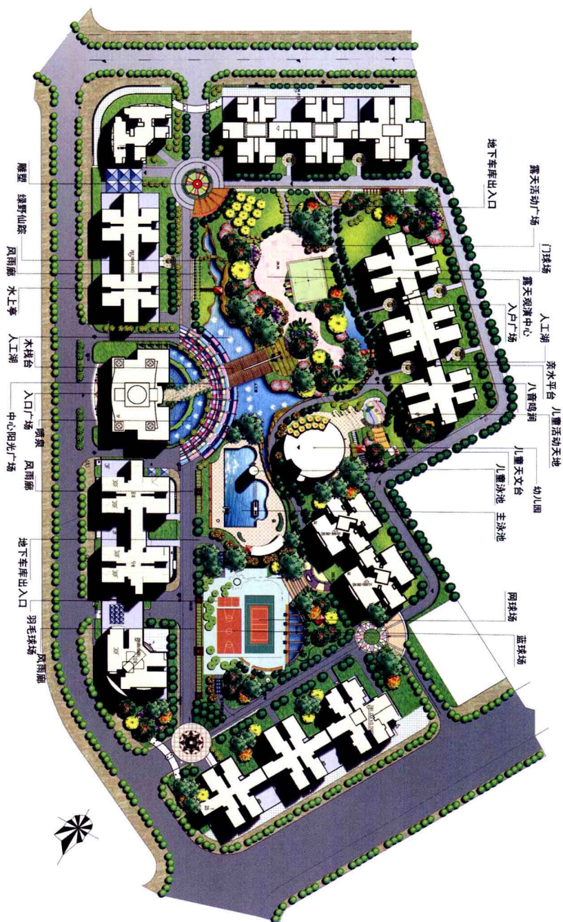
总平面图
