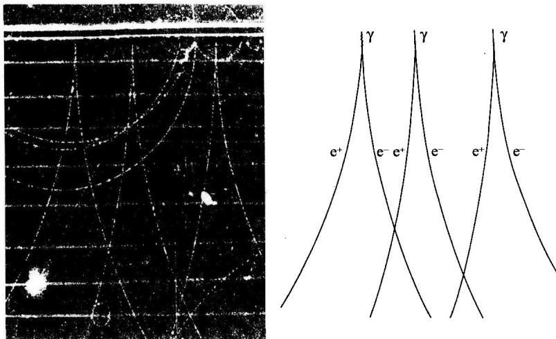
图 A.1 X 光的光子由上方入射, 经过铅板后, 产生电子-正电子对的径迹照片与分析图
