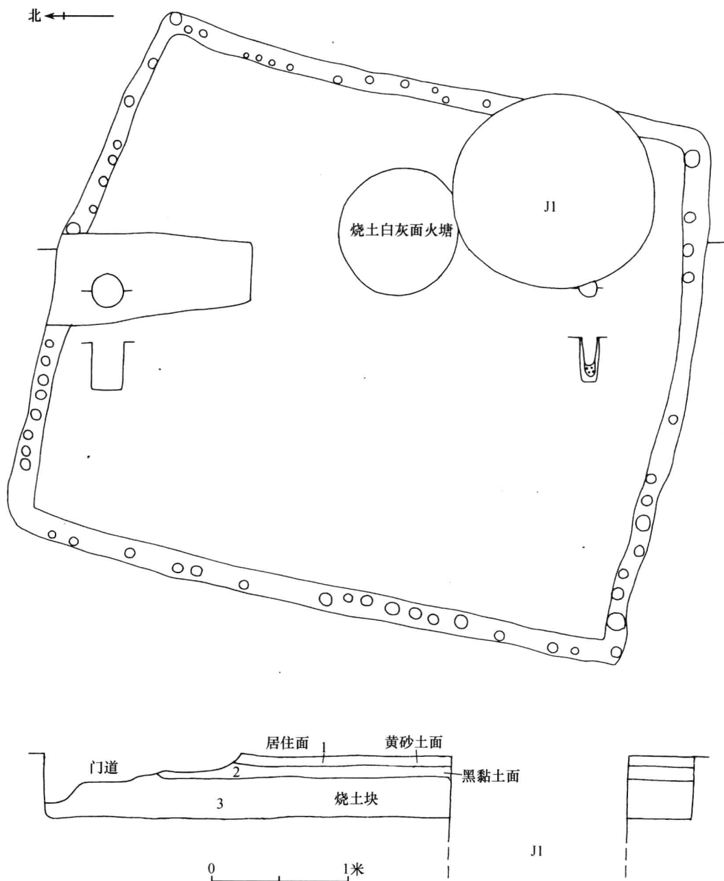
图三 F4 平、剖面图
