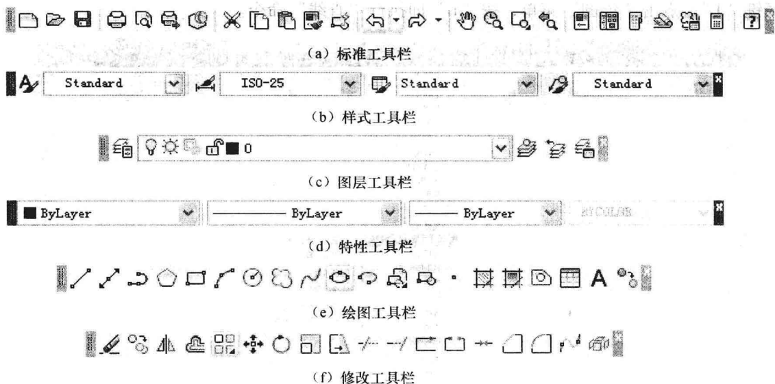
图 1-8 常用工具栏
