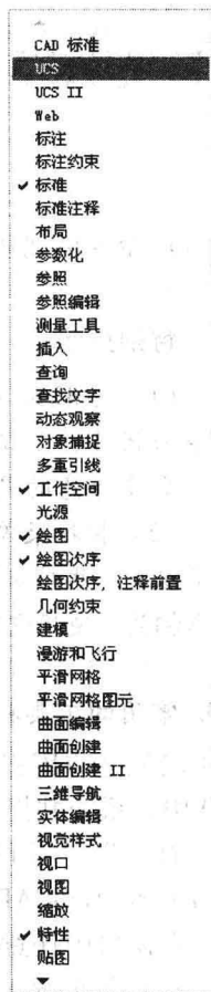
图 1-9 工具栏菜单
