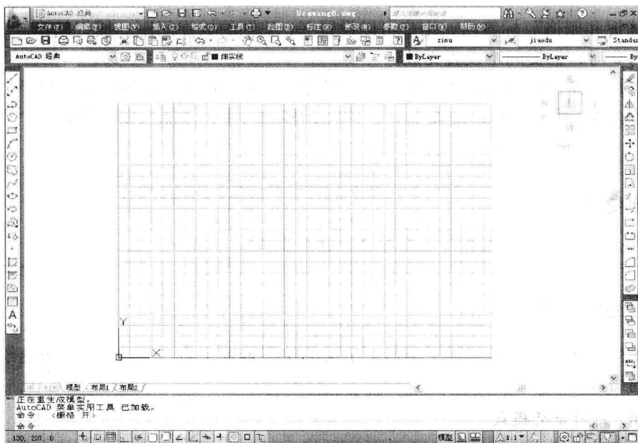
图 1-15 栅格
