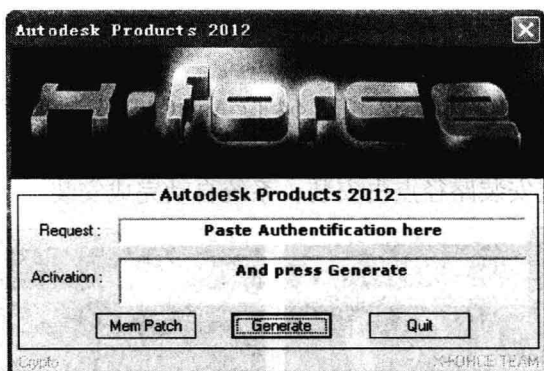
图 1-3 获取激活码
