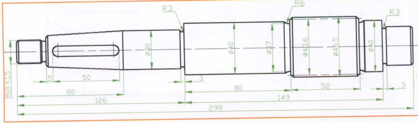
高速轴
