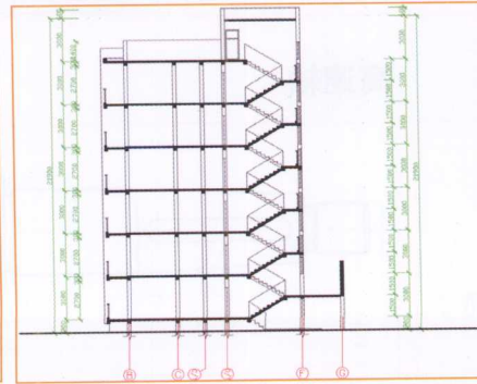
标注住宅剖面图
