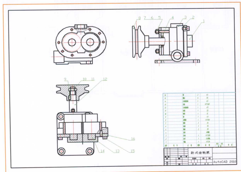
卧式齿轮泵
