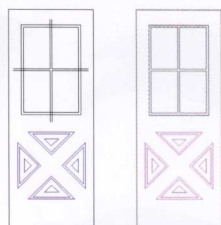
编辑多线
