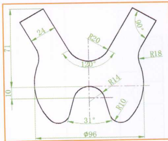
机械零件图 角度标注
