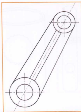
机械零件图 角度标注
