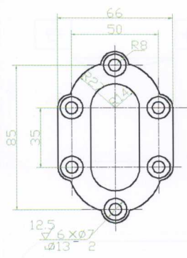
泵体零件图
