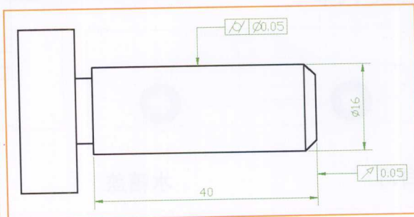
螺柱 形位公差标注
