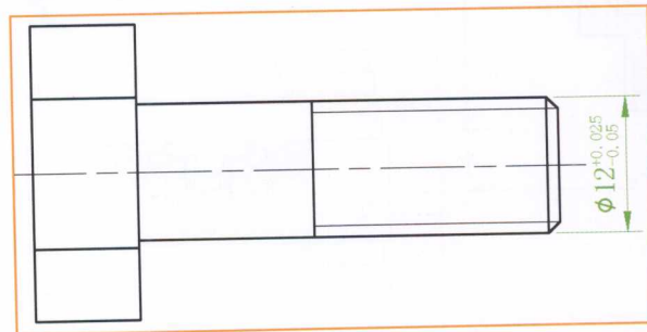
螺栓 公差标注
