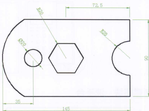
拔叉 折弯标注
