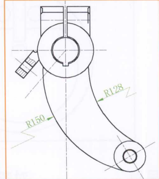
拔叉 折弯标注
