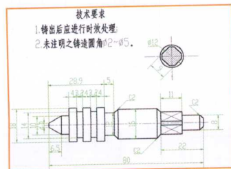
阀杆
