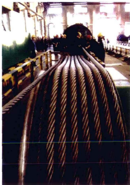
图为公司优质产品中国名牌「巨龙」牌钢丝绳生产现场
