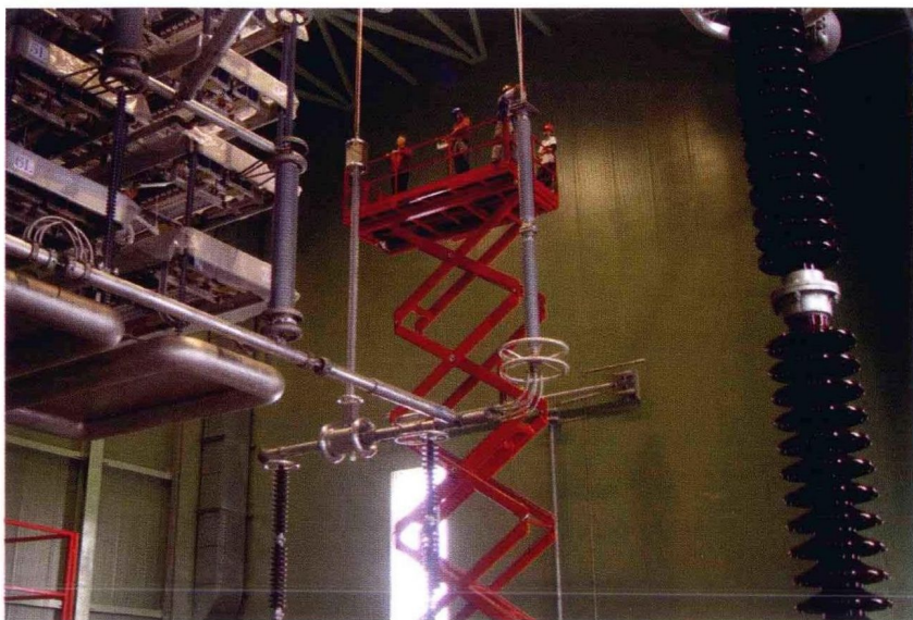
图为安顺换流站阀厅设备安装——光缆敷设现场
