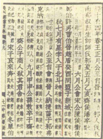
《春秋》中关于哈雷慧星的记载
