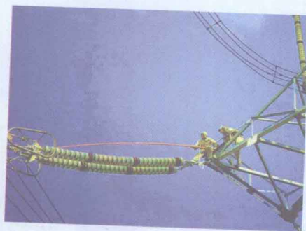
带电测量绝缘子零值
