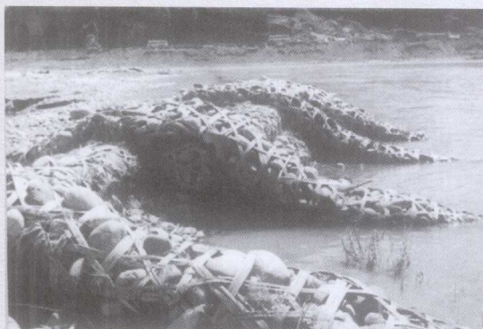
通济堰古拦河坝
