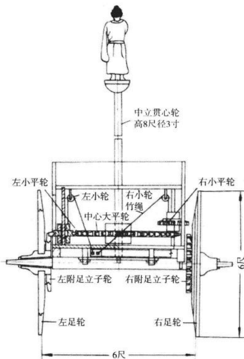
◆指南车原理图
