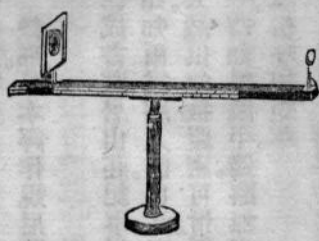
視力表
